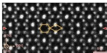
四酸化三鉄APBの電子顕微鏡像。走査透過型顕微鏡による高角度環状暗視野(HAADF-STEM)像([1-10]晶帯軸)
